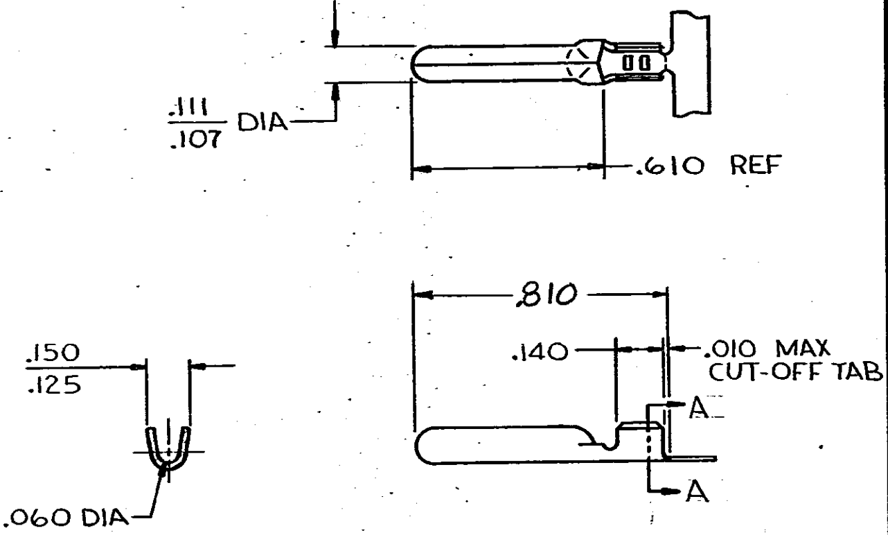
SECTION A-A
